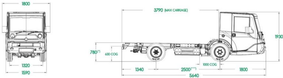
»eCarry«-Fahrgestell mit Niederflur-Fahrerhaus (Bild: Kanalreiniger.eu).
