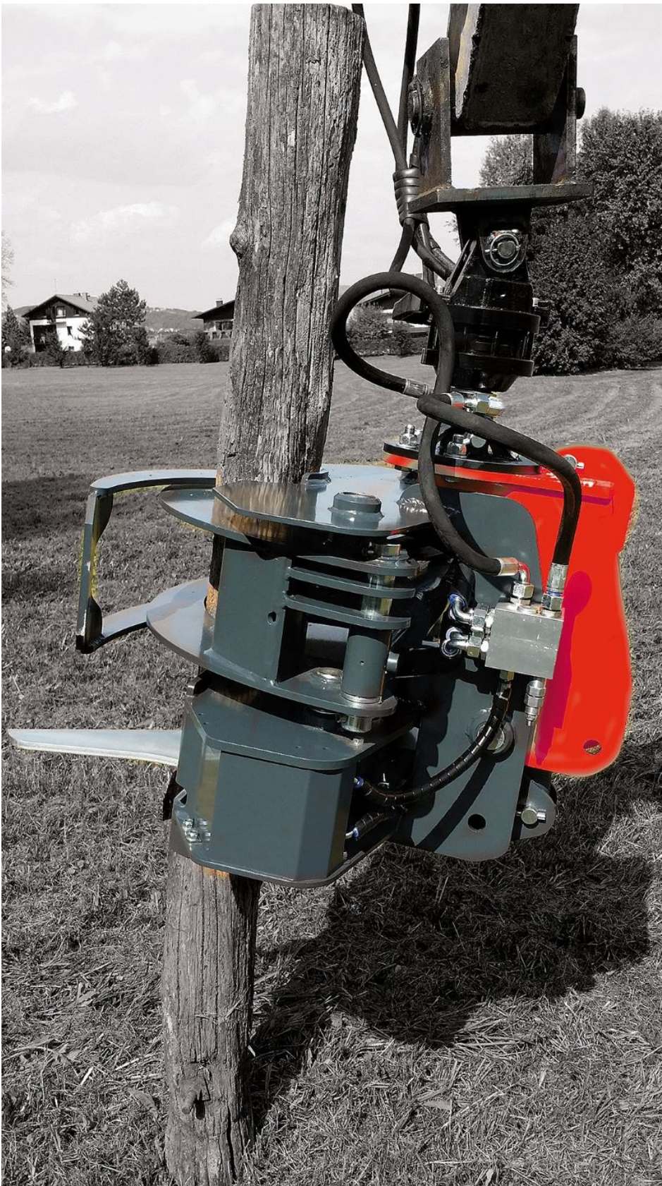
Ein Fällgreifer für den Bagger- und Krananbau (Bild: Beha).
